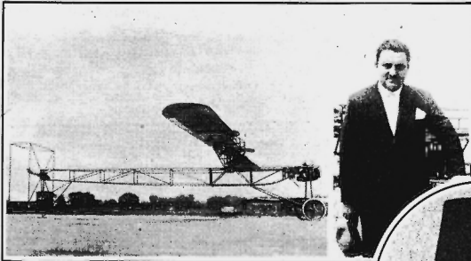
ALEMANIA. —El nuevo helicóptero, inventado en Berlín por el Ing. Zischka, que aparece a la derecha. Este aparato puede ascender y descender verticalmente. Las pruebas realizadas en el aeródromo de Tempelhofen han dado resultados alentadores.
