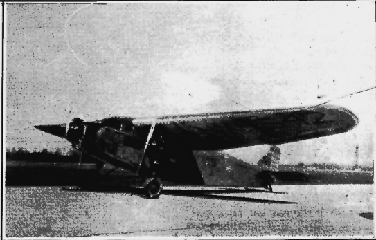
ESTADOS UNIDOS. —Monoplano Ford, de tres motores, enteramente construido de metal, que usará el Comandante Richard E. Byrd en su expedición al Polo Sur. Este avión ha sido expresamente construido para el vuelo al polo.
